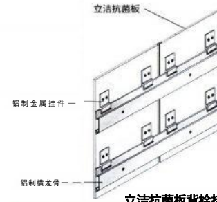
立洁抗菌板背栓挂装示意图
