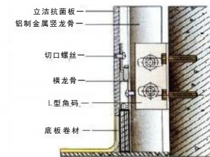
立洁抗菌板地面连接示意图
