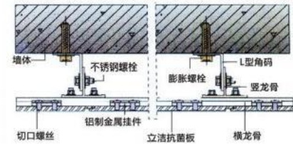
立洁抗菌板水平剖图
