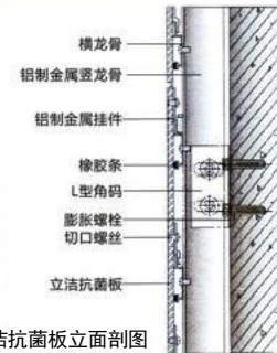
立洁抗菌板立面剖图
