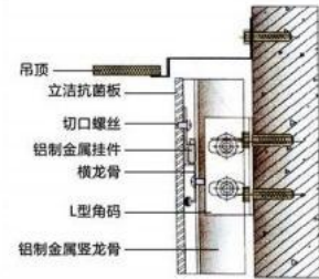
立洁抗菌板吊
