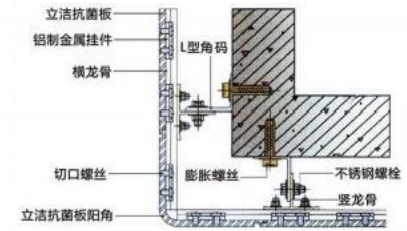
立洁抗菌板转角示意图
